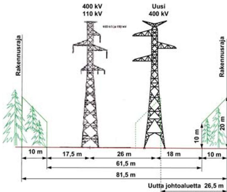
Kuvakaappauksessa voimajohtolinjakäytävien mitoitusesimerkki. Lähde: Pori Energia 2024 ja Fingridin ohje: Naapurina voimajohto.
